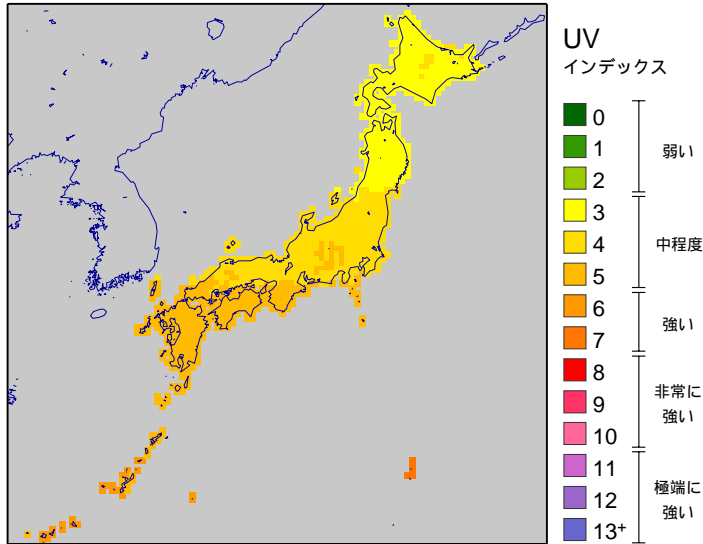
図1：4月の日最大UVインデックスの月平均分布(解析値)
