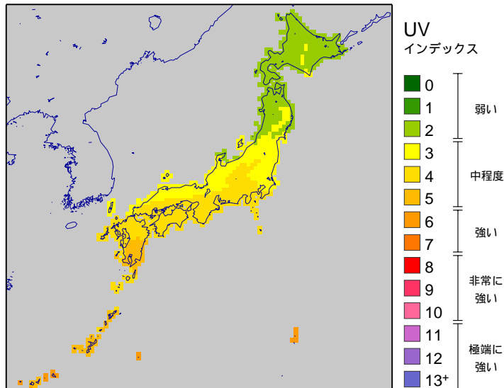
図1：3月の日最大UVインデックスの月平均分布(解析値)
