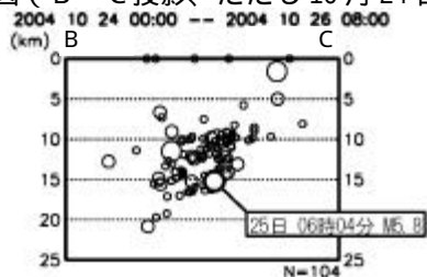
断面図（B - C 投影、ただし 10 月 24 日～）
