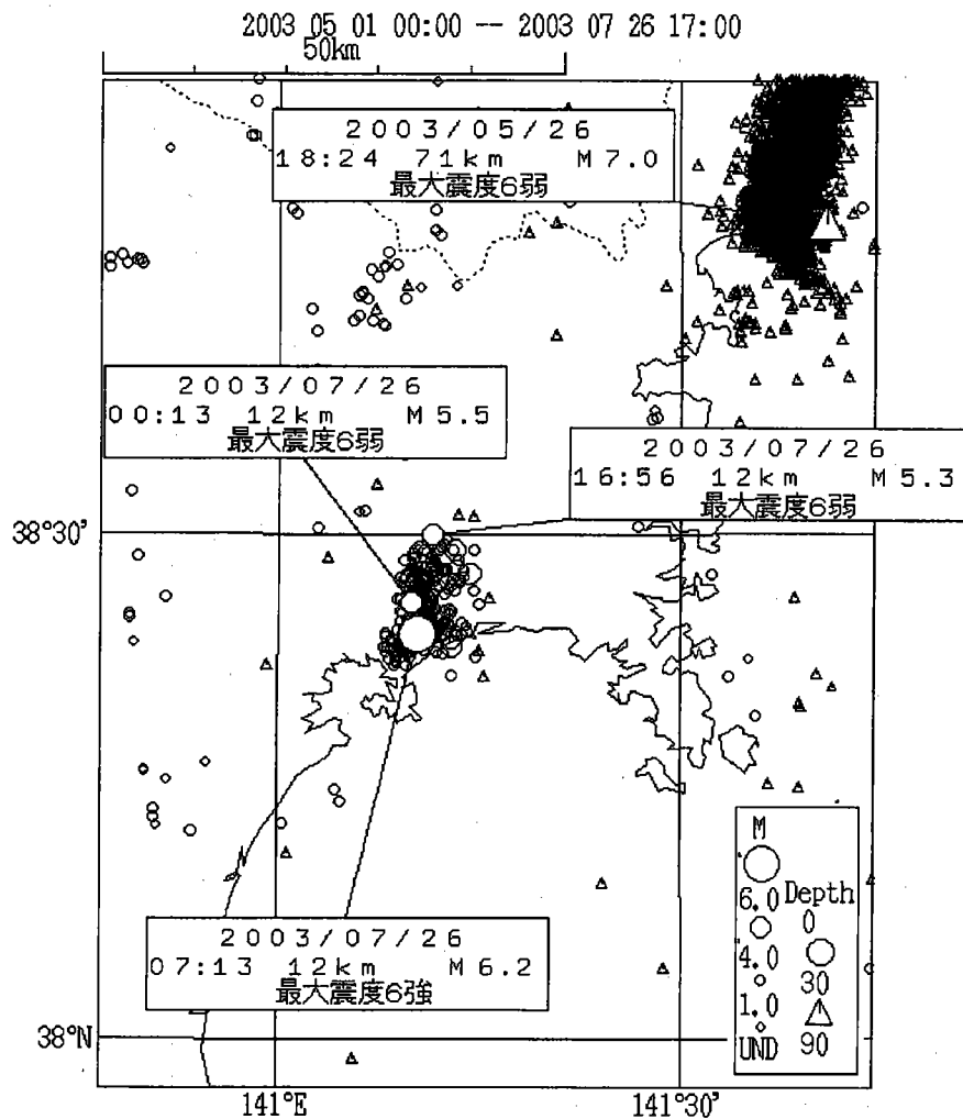
図1 震央分布図
