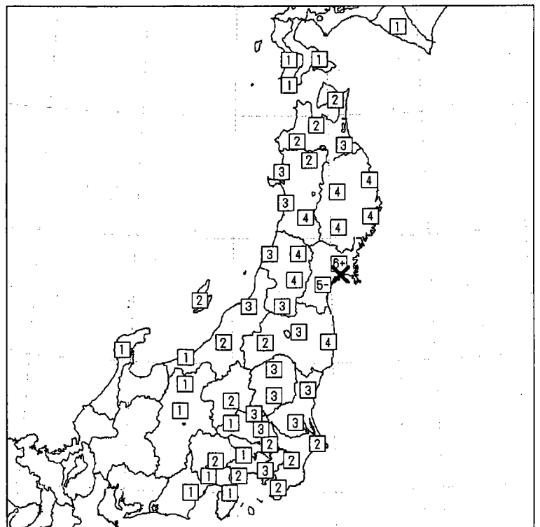
図 2 各地域の震度分布図
