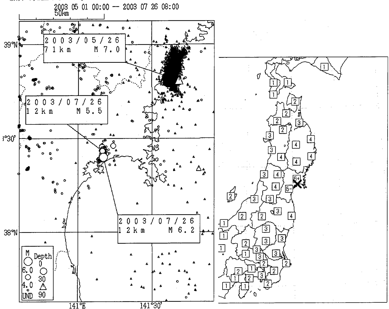
図1 震央分布図
