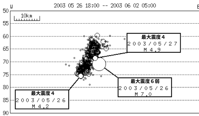
断面図
