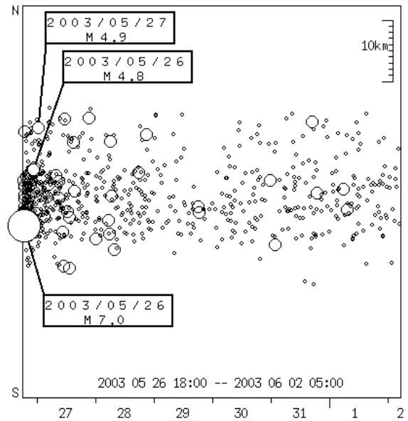
時空間分布図 (N-S 方向)
