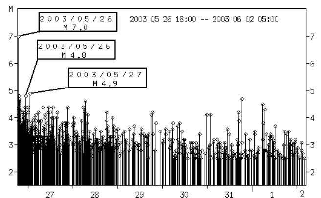
地震活動経過図
