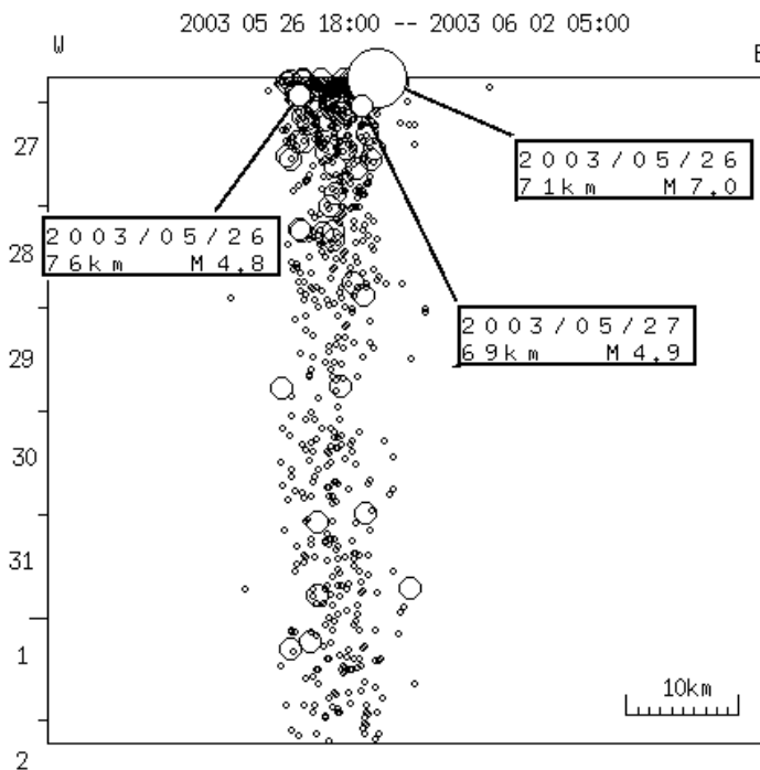
時空間分布図 (W-E 方向)
