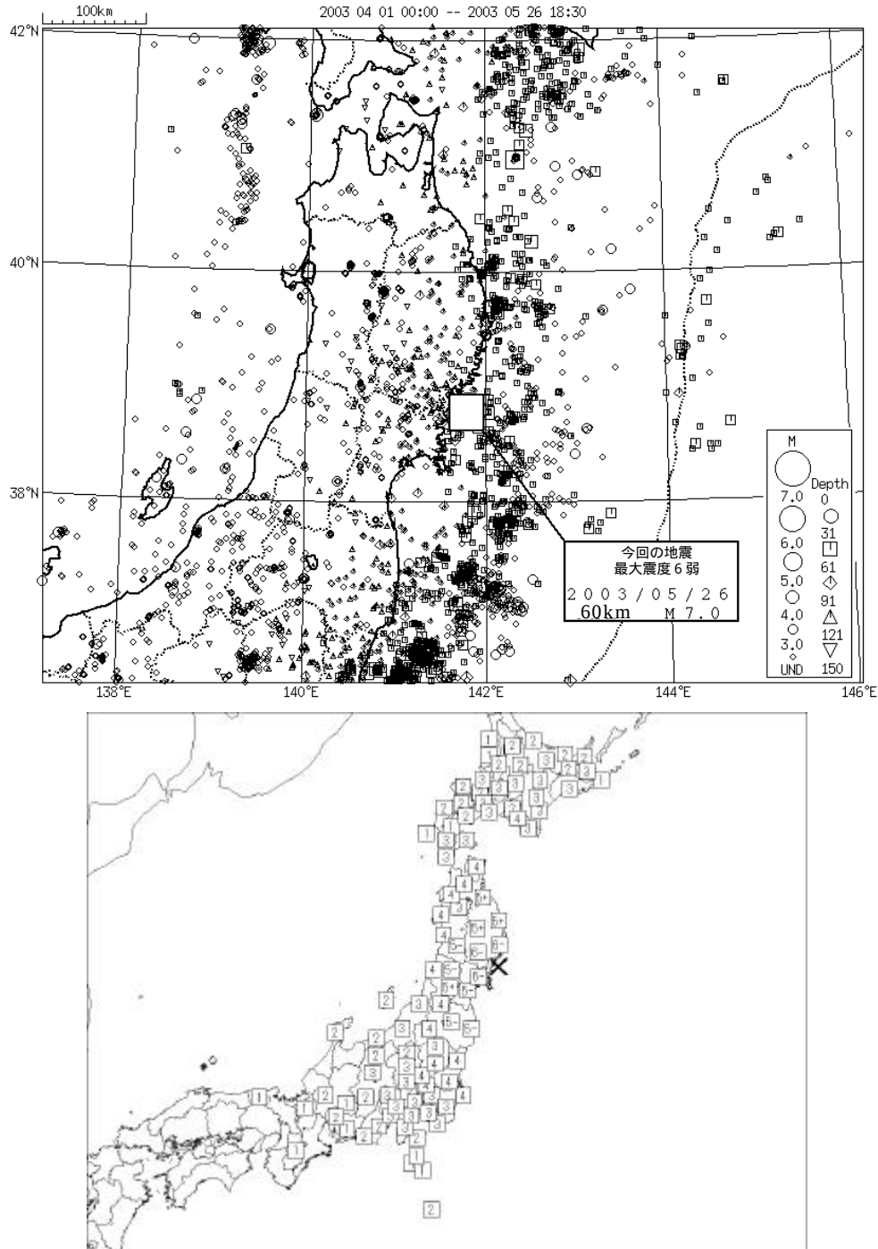
図 震央分布図および各地域の震度分布図 2003年4月1日～2003年5月26日18時30分
