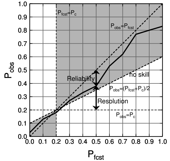
図 C.4.1 確率値別出現率図の模式図。横軸は予測現象出現確率、縦軸は実況現象出現相対頻度、実線が信頼度曲線である。対角線、直線 P_{obs} = P_c との差の二乗がそれぞれ信頼度 (Reliability)、分離度 (Resolution) への寄与に対応している。灰色の領域内の点はブライアスキルスコアに正の寄与を持つ。
