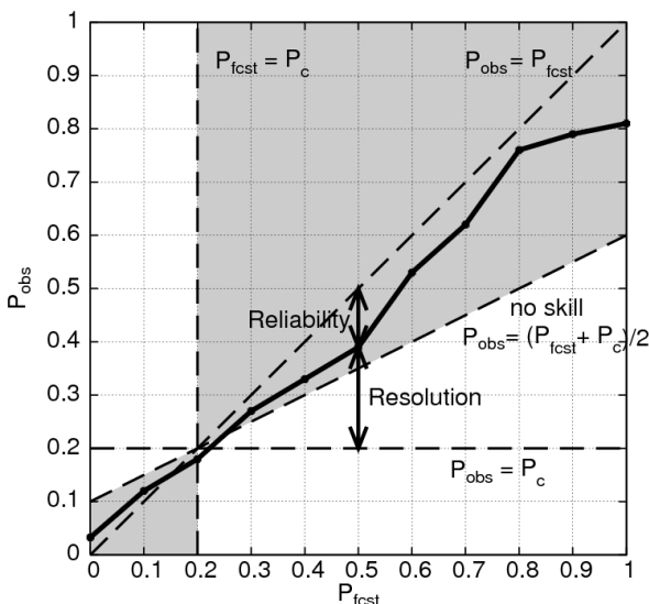
図B.4.1 確率値別出現率図の模式図。横軸は予報現象出現確率、縦軸は実況現象出現相対頻度、実線が信頼度曲線である。対角線、直線 P_{obs} = P_c との差の二乗がそれぞれ信頼度 (Reliability)、分離度 (Resolution) への寄与に対応している。灰色の領域内の点はブライアスキルスコアに正の寄与を持つ。
