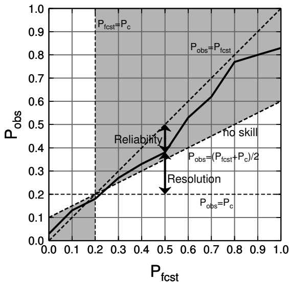
図 A.4.1 確率値別出現率図の模式図。横軸は予測現象出現確率、縦軸は実況現象出現相対頻度、実線が信頼度曲線である。対角線、直線 P_{obs} = P_c との差の二乗がそれぞれ信頼度 (Reliability)、分離度 (Resolution) への寄与に対応している。灰色の領域内の点はブライアスキルスコアに正の寄与を持つ。
