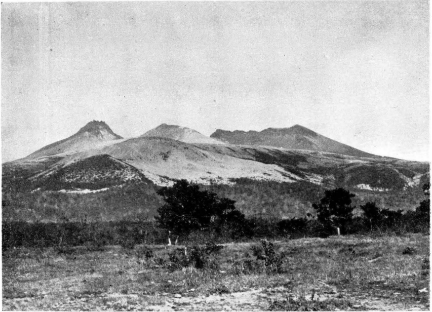
第一圖 噴火前に於ける駒ヶ嶽の外貌
