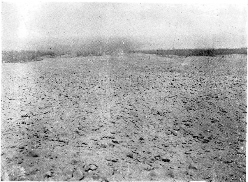
る流に岸海突破を林樹の流塊石野燒 圖五十第 (撮本根日一十二月六)
