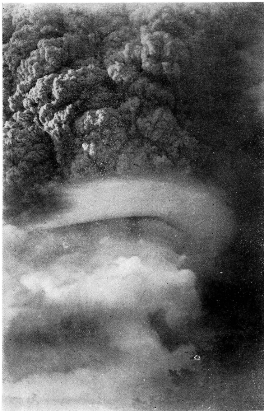
（攝氏丸松校學範師館函分五十二時八日七十月六）雲狀環るたれは現に邊周煙噴 圖 九 第
